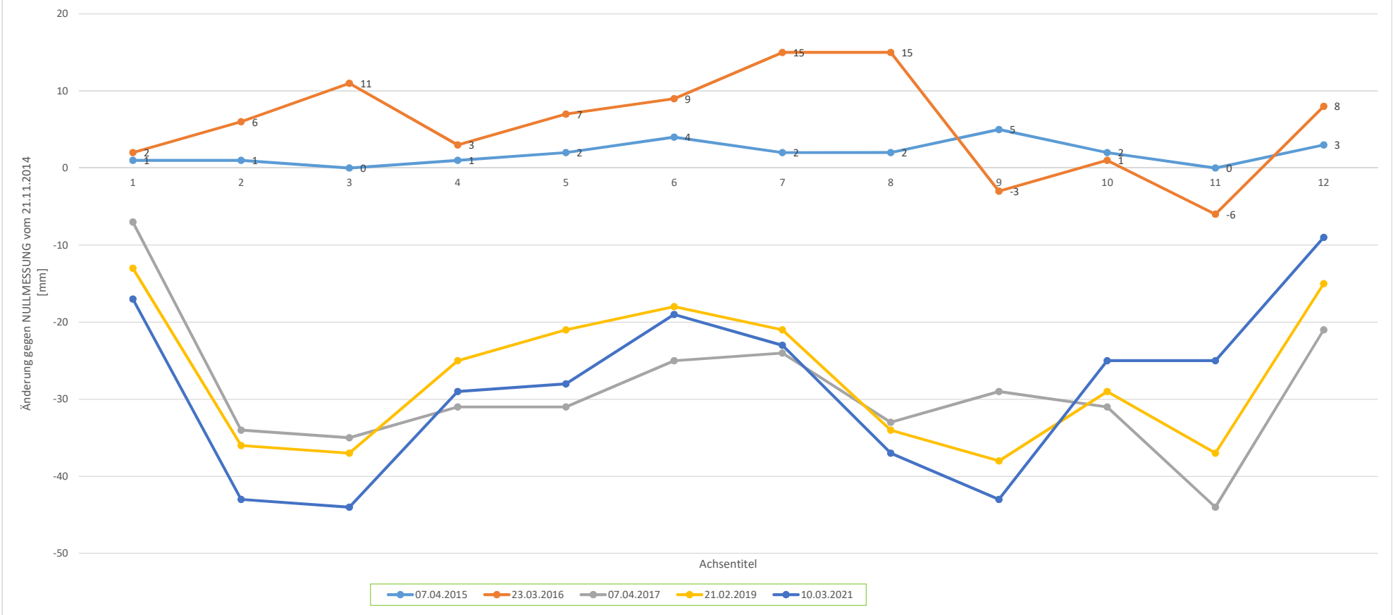
DEFOMATIONSMESSUNGEN DEPONIE HOHLER STEIN HÖHENÄNDERUNG_2015-2021
